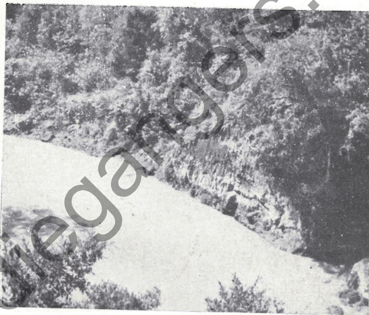
De Tji Sokan nabij Tjirandjang , heeft een smalle diepe kloof uitgesleten
